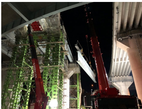
＜橋梁桁架設＞
